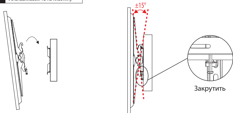
Шаг 3 Устанавливаем ТВ на пластину
