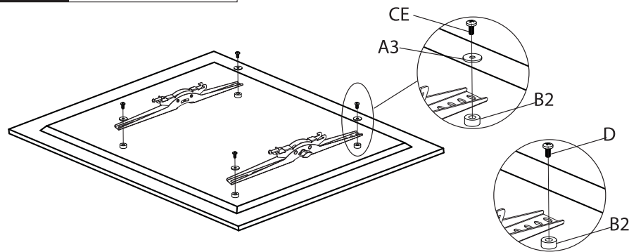
Шаг 2 Установка кронштейна на ТВ
